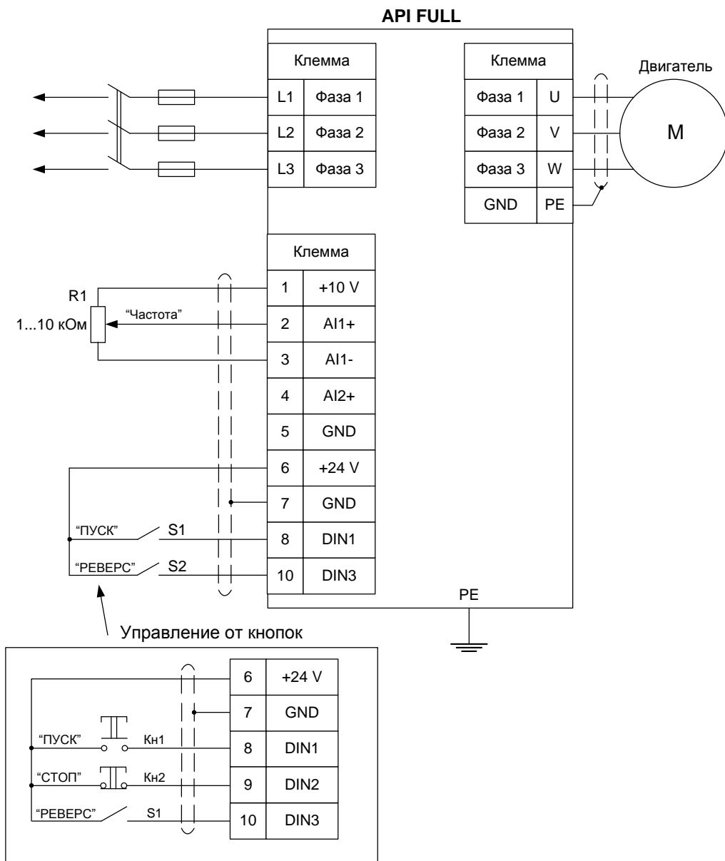
Рисунок 1 – Схема подключения к клеммам преобразователя частоты Vascon 10
