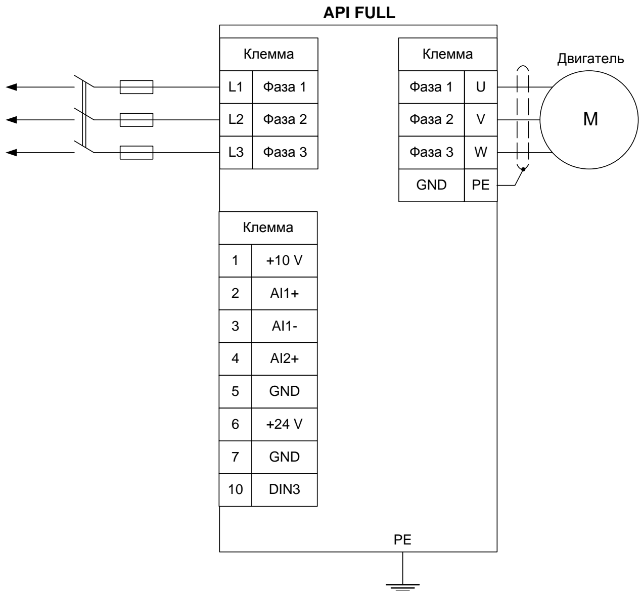
Рисунок 3 – Схема подключения к клеммам преобразователя частоты Vacon 10
