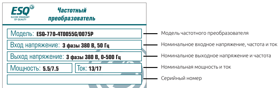
Рисунок 2-4. Изображение шильды частотного преобразователя ESQ-770
