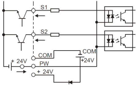
Внешнее питание (NPN режим)
