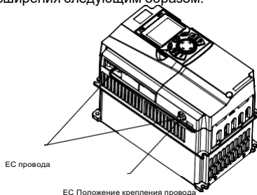
Рис А.5 Прокладка проводов для платы расширения
