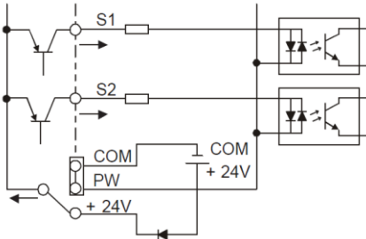
Внутреннее питание (PNP режим)
