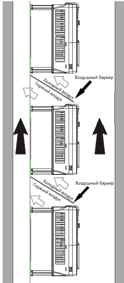
Рис 4.5 Вертикальная установка
