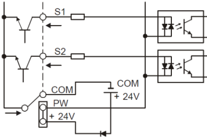
Внутреннее питание (NPN режим)
