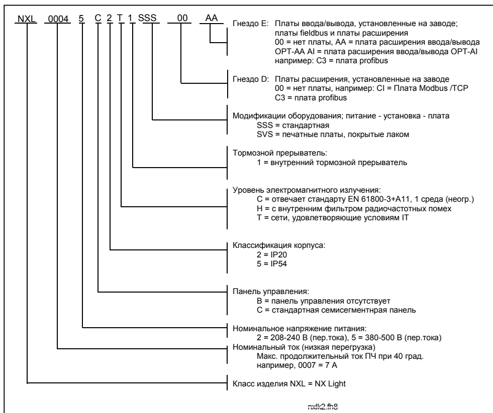
Рис. 3-2. Расшифровка кода условного обозначения Vacon NXL для типоразмеров MF4 - MF6.
