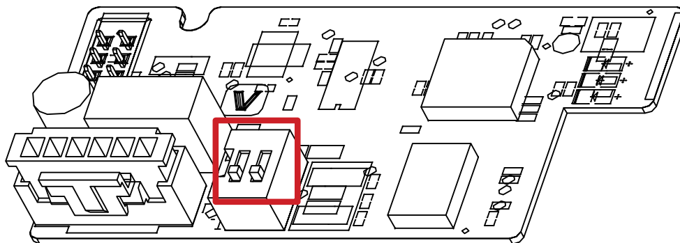
Рис. 4. Переключатель терминатора
