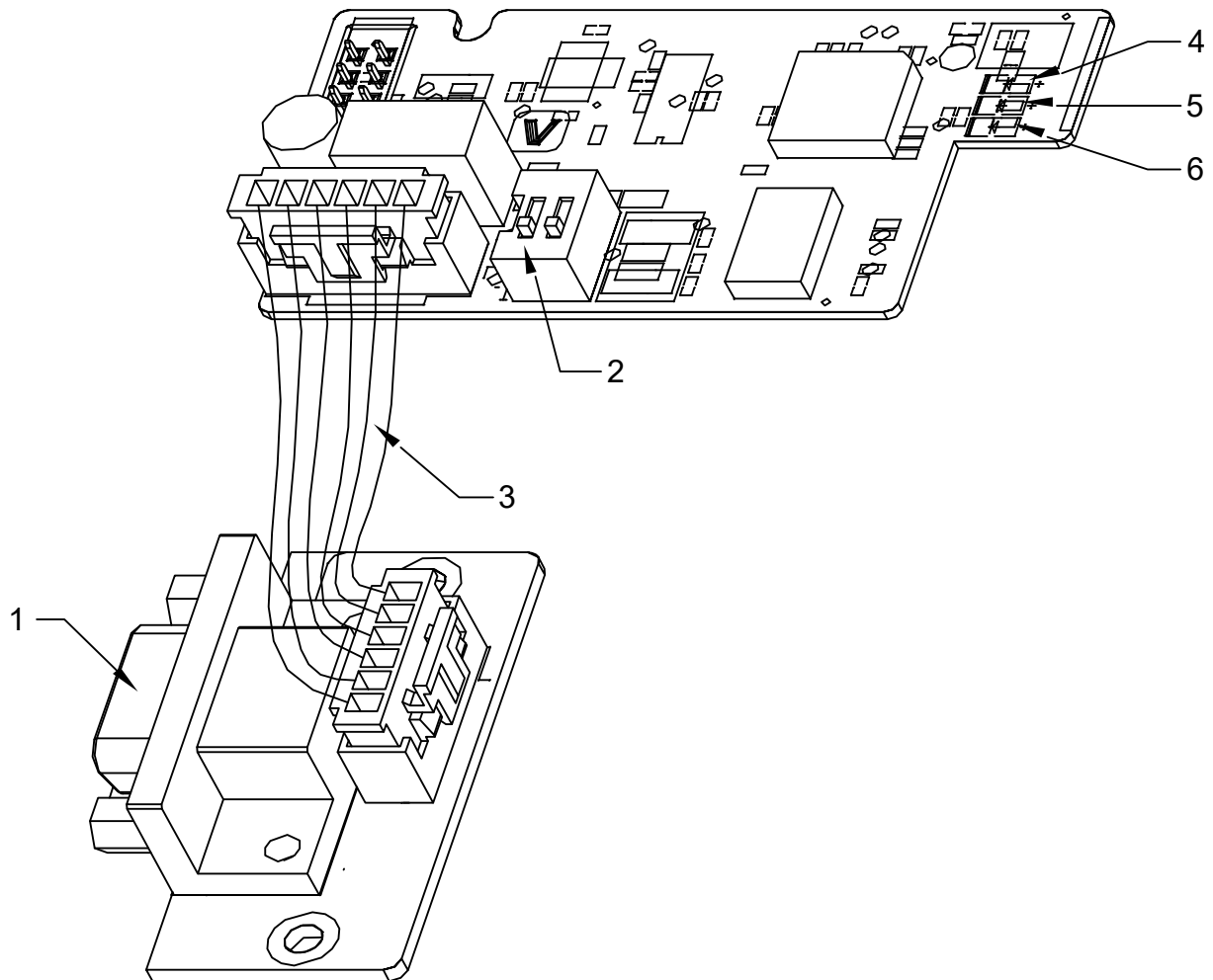
Рис. 1. Интерфейс Profibus
